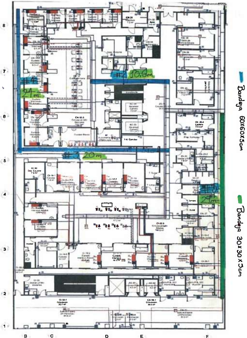
Piso 3 Bandeja electrica 60x60x5cm y 30x30x5cm
