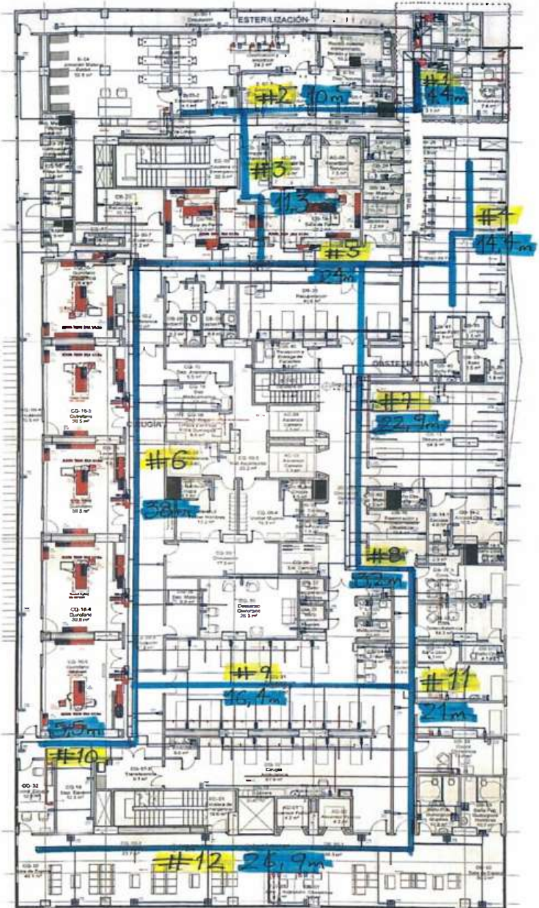
(d) PLANO DESCRIPTIVO DE LA MEMORIA
