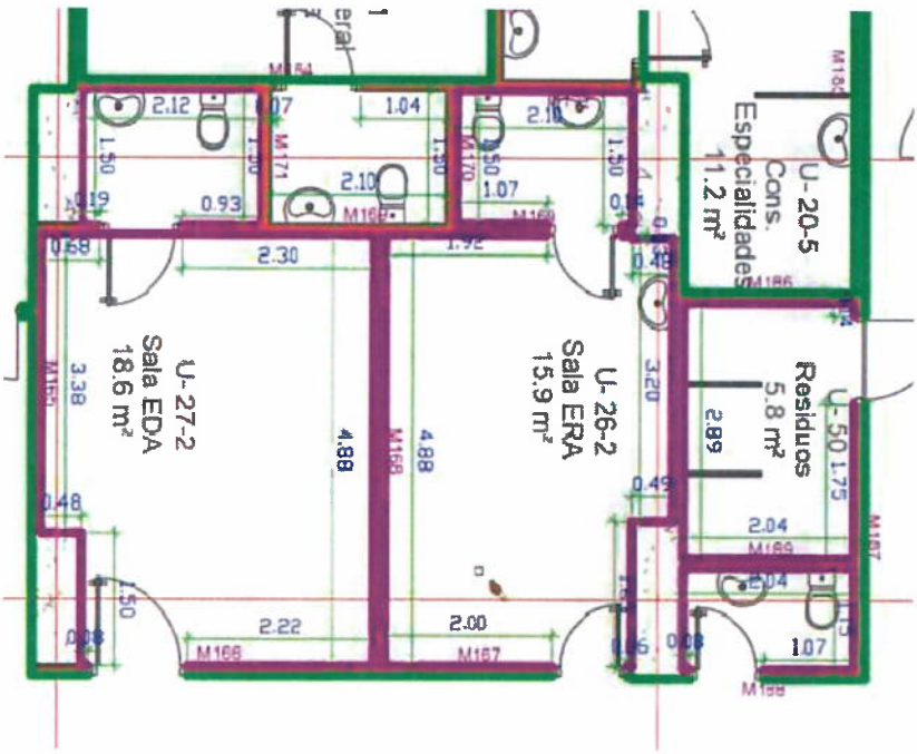
EJE D-E ENTRE 7-9
