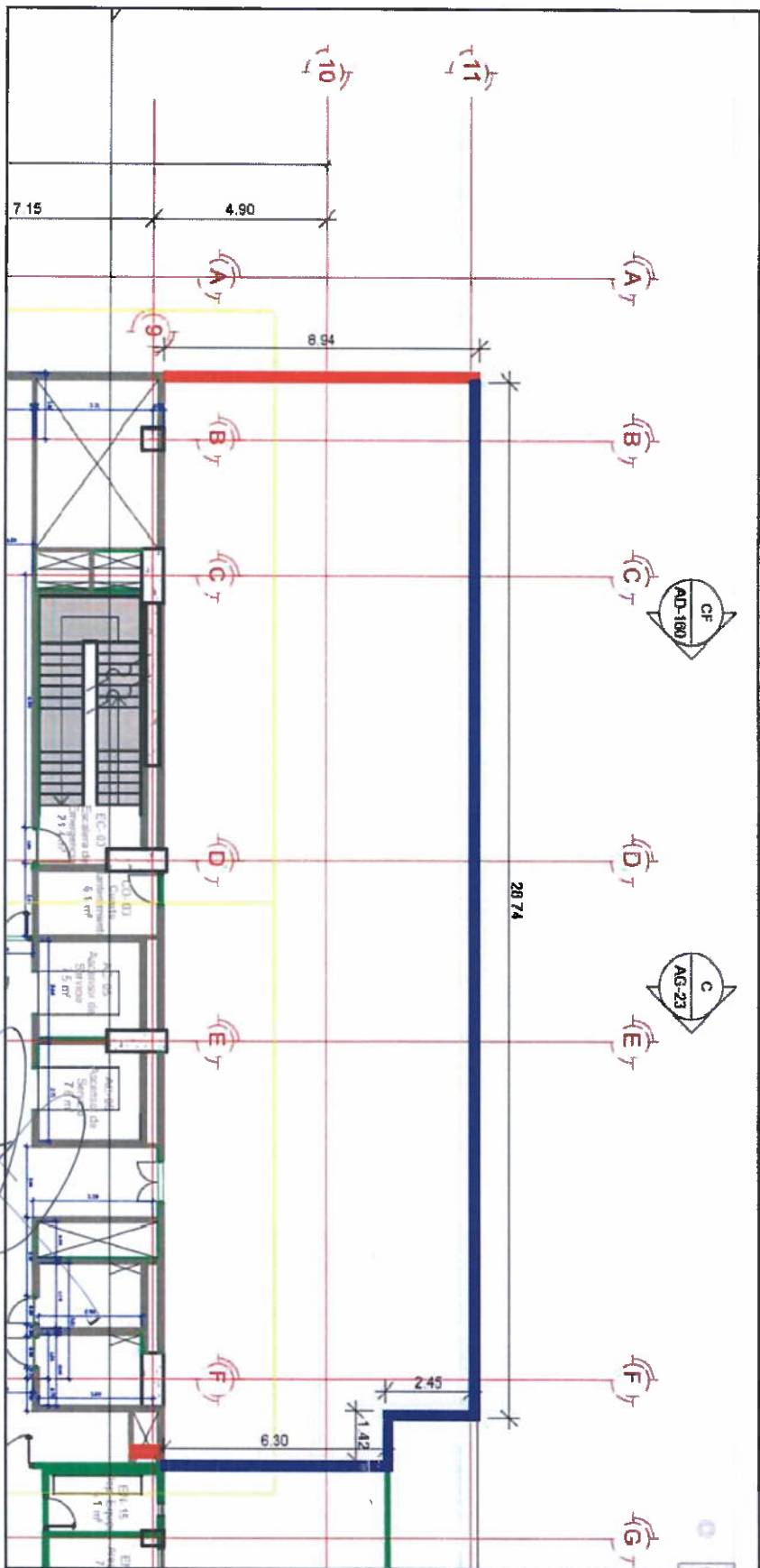
(d) PLANO DESCRIPTIVO DE LA MEMORIA - PISO 3
