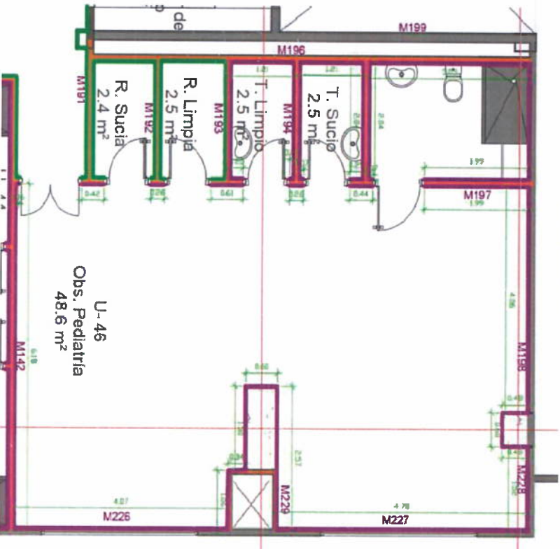
EJE E-F ENTRE 10-6
