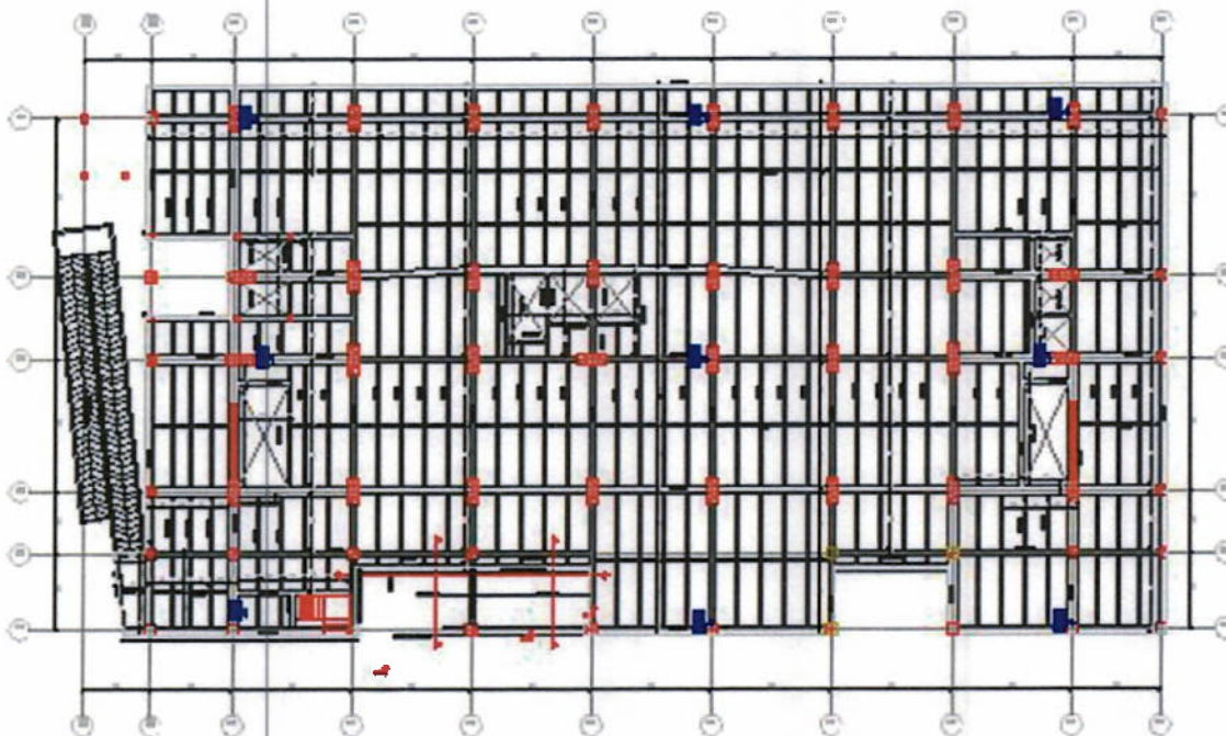
Ilustración 24. Puntos de control asentamientos
