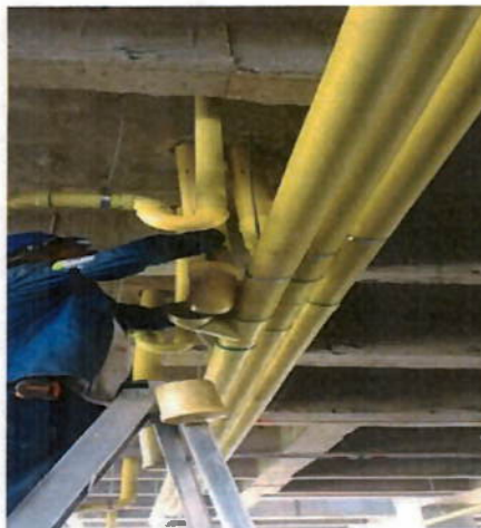
Ilustración 13. Descuelgue y tendido de red sanitaria bajo placa piso 3.
