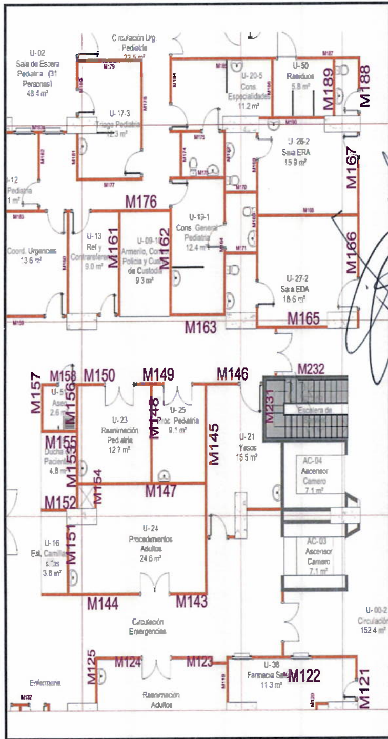
(d) PLANO DESCRIPTIVO DE LA MEMORIA PLANIMETRIA PISO 1
