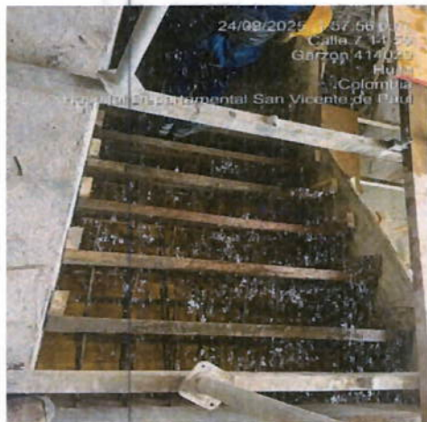
Ilustración 22 Armado de áceros
