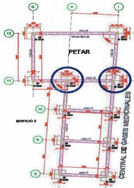
Ilustración 30 Planta de Cimentación Edificio 3 Lote B
