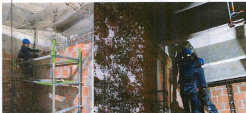
Ilustración 5 Armado de mampostería
